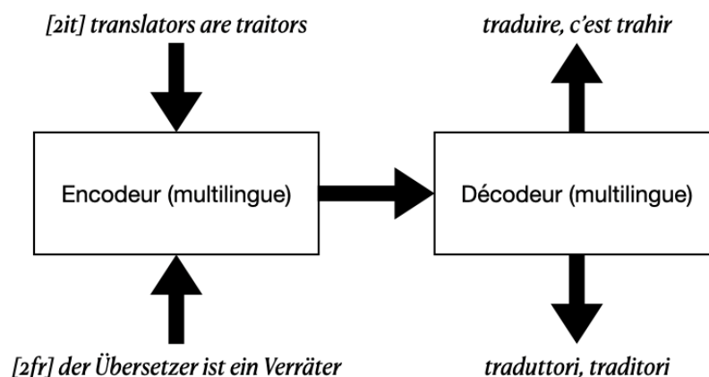
Figure 4. Une illustration de l'architecture encodeur-décodeur pour un système multilingue, comprenant un encodeur multilingue et un décodeur multilingue. Ce système traduit 4 couples de langues.
