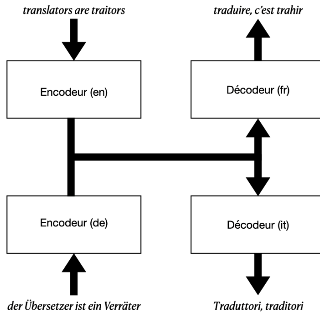
Figure 3. Une illustration de l'architecture encodeur-décodeur pour un système multisource-multicible, comprenant deux encodeurs et deux décodeurs. Ce système unique produit des traductions automatiques pour 4 couples de langues
