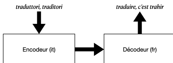
Figure 1. Une schématisation de l'architecture encodeur-décodeur d'un système bilingue. Encodeur et décodeur ne prennent en charge qu'une langue : l'italien en source, le français en cible.
