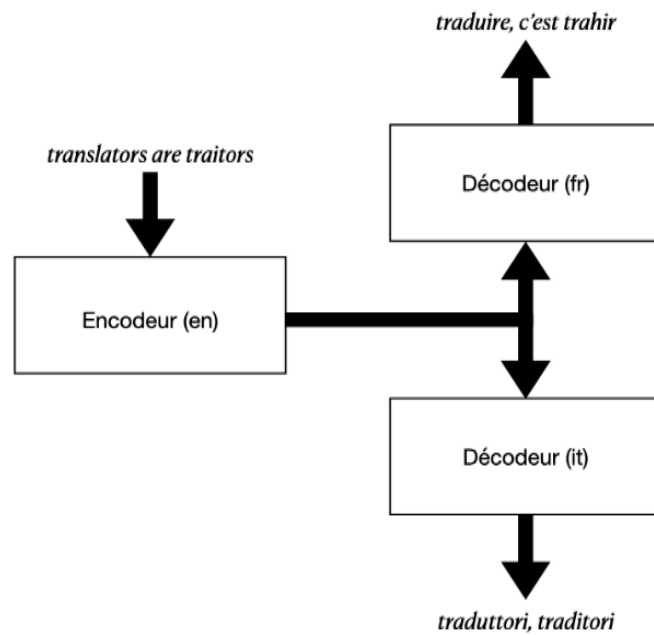
Figure 2. Une illustration de l'architecture encodeur-décodeur pour un système multilingue, comprenant un unique encodeur et deux décodeurs. Chaque décodeur ne prend en charge qu'une langue.
