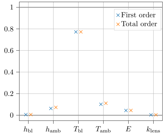
(d) Output T_C .
