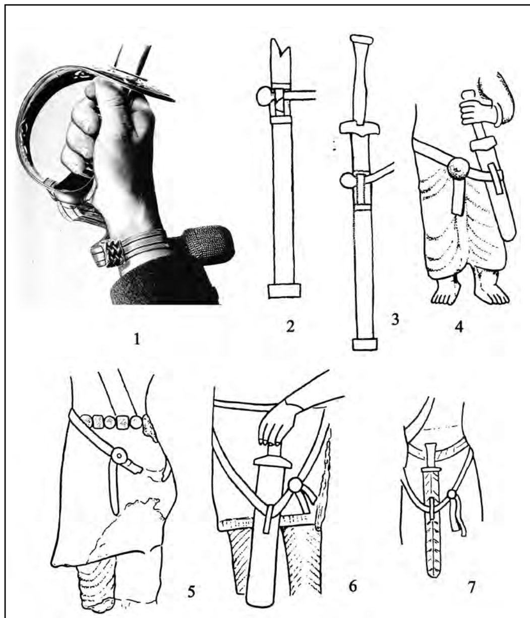
Рис. 5. Темляки (1) и фиксаторы португейных ремней на античном Среднем Востоке (2–7) 1 – вооружение шведской кавалерии 1943 г.; 2, 3 – Орлат; 4 – Шоторак; 5 – статуя кушанского царя; 6 – Хадда; 7 – Гандхара
