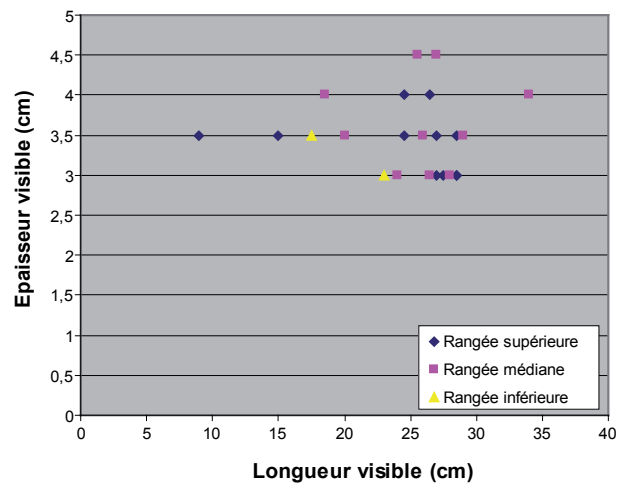
Figure 14 - Diagramme rapportant les mesures des terres cuites mises en oeuvre dans le parement du mur MR 32
