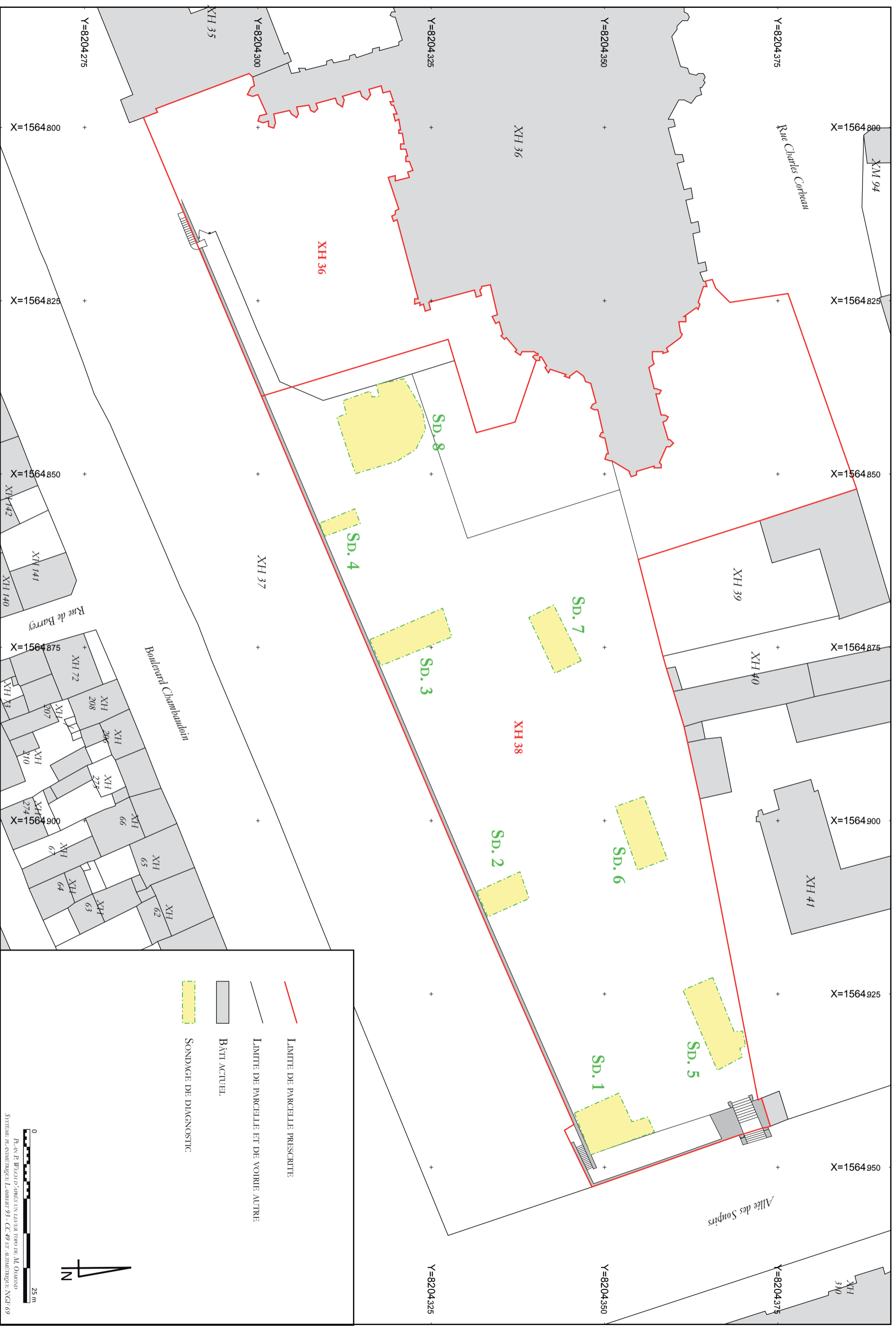
Figure 10 - Implantation et numérotation des sondages réalisés lors du diagnostic
