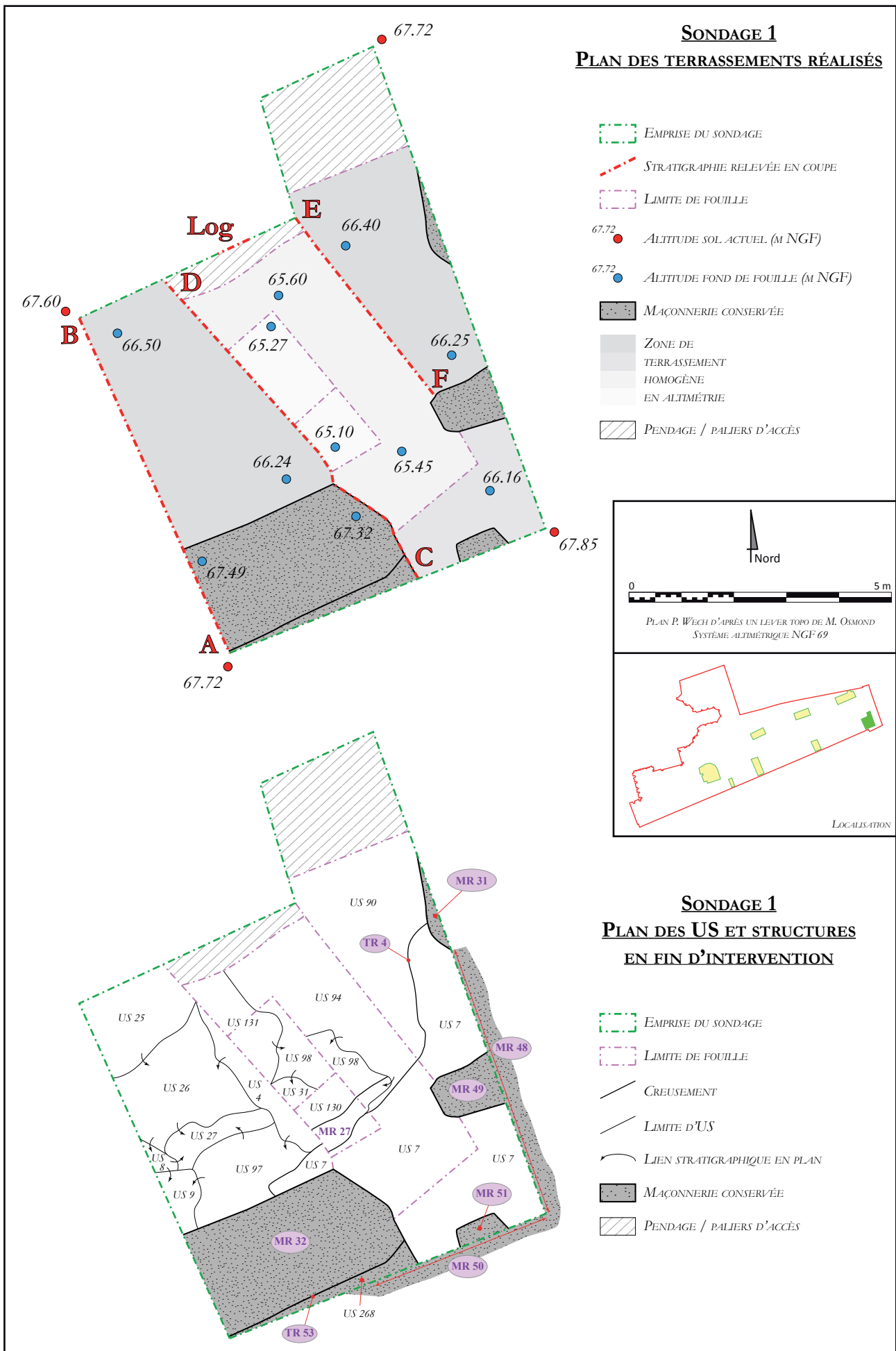
Figure 11 - Plan détaillé du sondage 1
