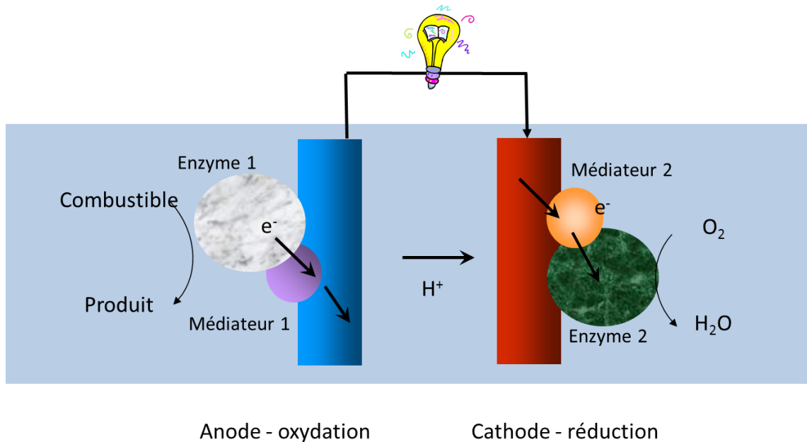
Figure 2 : Schéma simplifié d'une biopile enzymatique.
