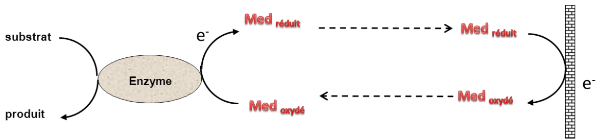
Figure 1 : Principe de la connexion électronique entre une enzyme et une électrode via un médiateur (Med) électrochimique.
