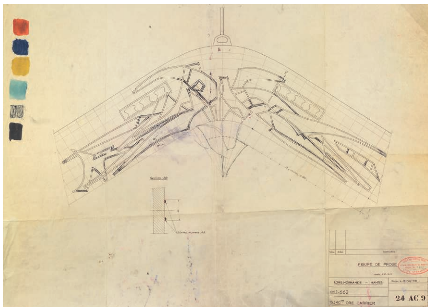
Fig. 15 – Plan technique et nuancier pour la figure de proue du Brissac
