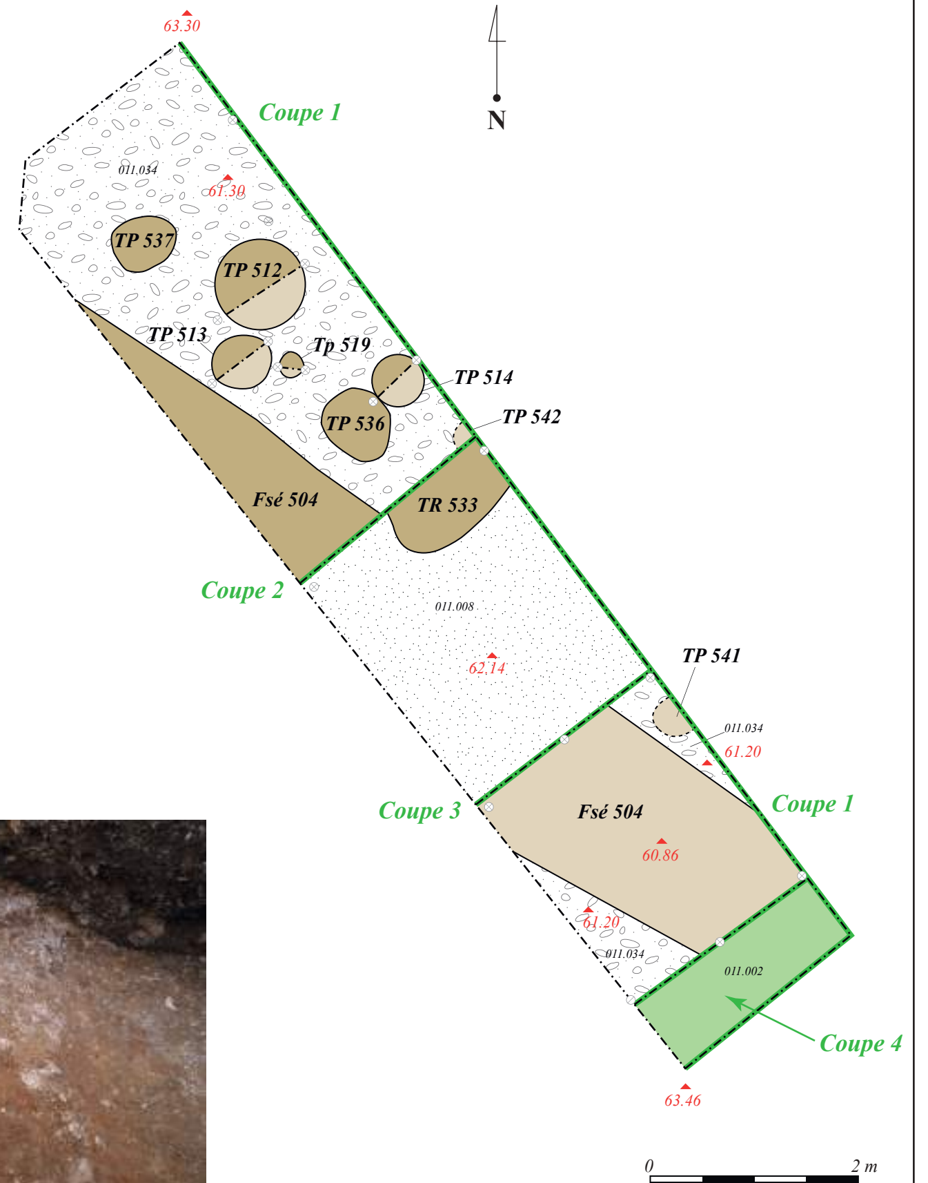
Planche 1 Sondage 11 - Plan général en fin de fouille
