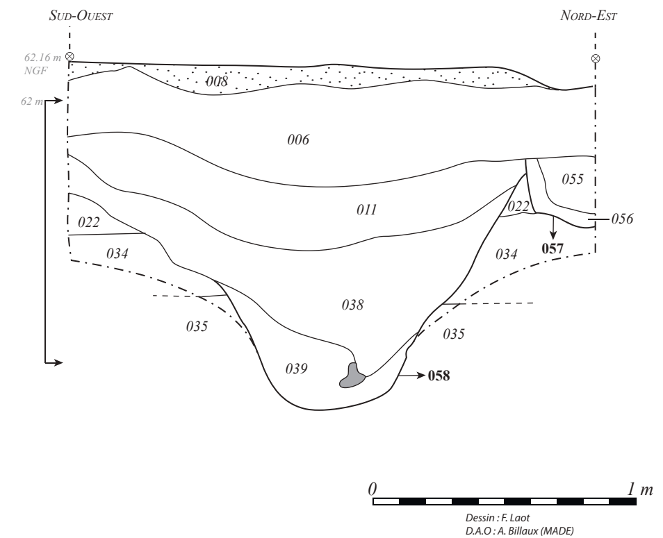
COUPE 3 : SUD-OUEST / NORD-EST
