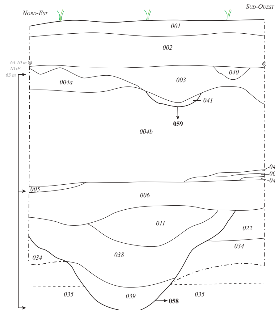
COUPE 4 : NORD-EST / SUD-OUEST
