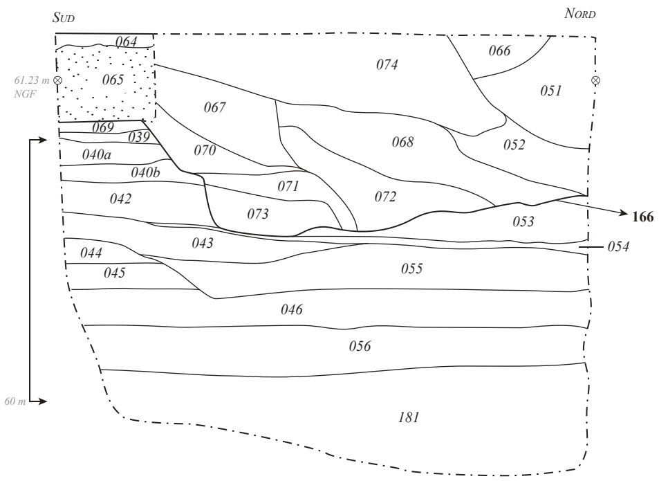
COUPE 6 : PARTIE EST / COUPE OUEST
