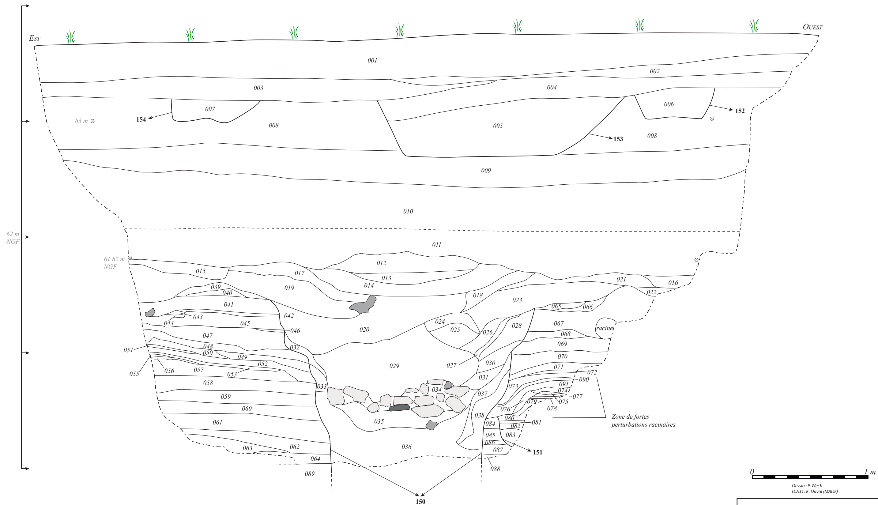
Planche 66 Sondage 41 - Coupe 1
