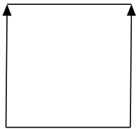
Figura 1. El diagrama topológico correspondiente a un cilindro.
