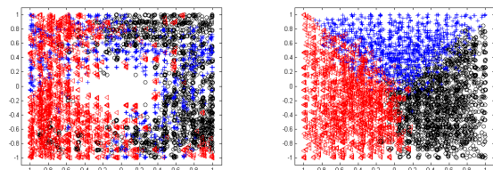
(a) Classifieur A (b) Classifieur B
