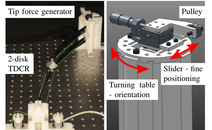
(d) Setup for tip stiffness measurement.
