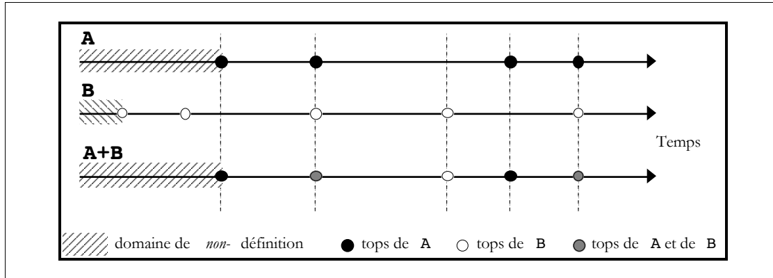
Figure II.5 : Domaine de définition et horloge d'une expression arithmétique entre deux streams, en fonction des domaines de définition et des horloges des streams arguments.
