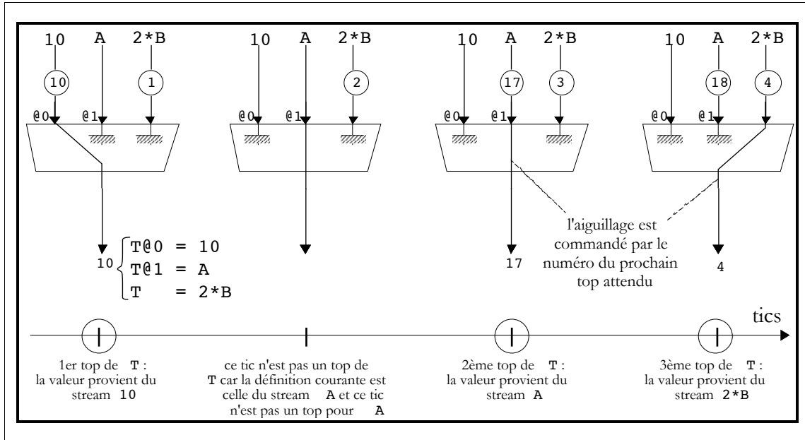
Figure II.6 : La définition quantifiée des streams représentée comme un aiguillage entre différents streams. Les valeurs d'un stream en un top sont représentées comme des jetons circulant sur des arcs. Une définition quantifiée permet de choisir de quelle équation (i.e. de quel arc) proviendra la valeur au prochain top du stream. Ce choix dépend du numéro du prochain top attendu. On ne passe d'une équation de définition à une autre, que quand un top s'est produit pour le stream défini par l'équation courante. Par exemple, au deuxième tic, l'équation courante est celle qui définit le stream T comme étant égal au stream A. Ce tic n'est pas un top de A et par suite, cette équation reste l'équation de définition courante de T jusqu'à ce qu'un top proviennent de A et déclenche le changement de définition.
