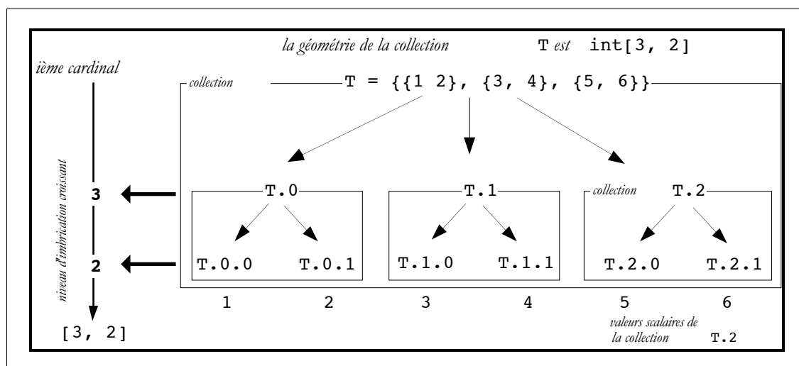
Figure III.4 : La géométrie des collections imbriquées homogènes de 81/2.
