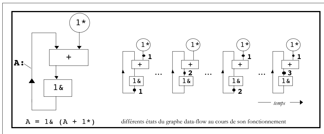
Figure V.5 : Graphe d'un compteur data-flow (à gauche) et son fonctionnement (à droite). Les jetons sont figurés par des pastilles sur les arcs. Le nœud 1^* est un générateur de « 1 » et le nœud 1\& génère le jeton « 1 » puis transmet à sa sortie les jetons qui se présentent en entrée. La suite des jetons qui passent sur l'arc A est la suite des entiers strictement positifs.
