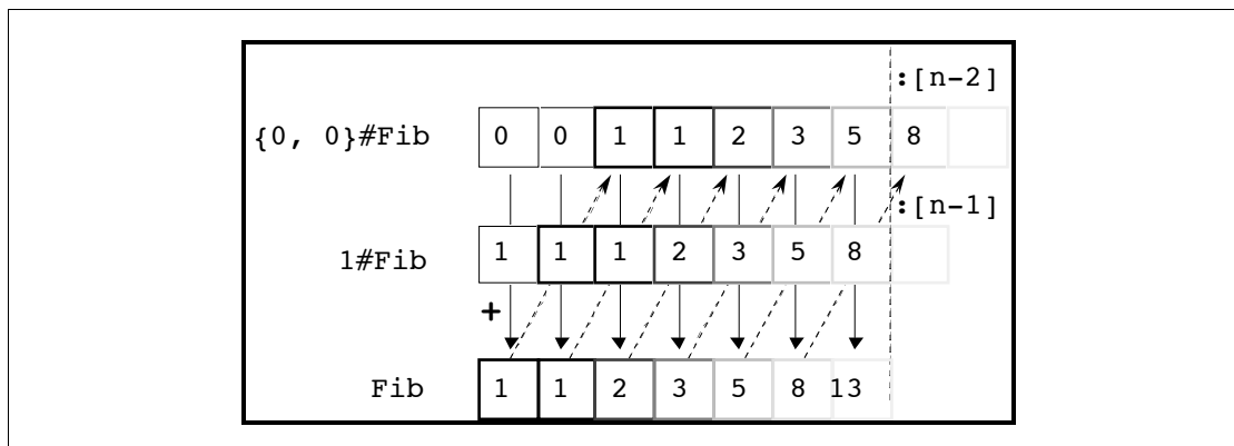
Figure III.11 : Expression récursive de la collection Fib (son i ème élément a pour valeur la valeur du i ème élément de la suite de Fibonacci commençant par 0 et 1). Chaque ligne représente une sous-expression de la définition de Fib . Les flèches représentent des dépendances entre les éléments des collections. Une flèche verticale correspond à une dépendance entre deux éléments de même indice. La concaténation introduit un décalage vers la droite et cette translation des valeurs est figurée par les flèches obliques. La barre verticale indique la troncature des collections. Les différents niveaux de gris indiquent, du plus sombre au plus clair, l'ordre d'évaluation des éléments.
