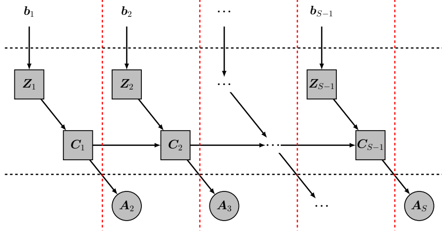
FIGURE 3 – Relation séquentielle entre les variables au fil du trajet : les variables latentes sont indiquées dans des carrés, tandis que les variables observées sont dans des disques ; les traits verticaux rouges séparent les gares.
