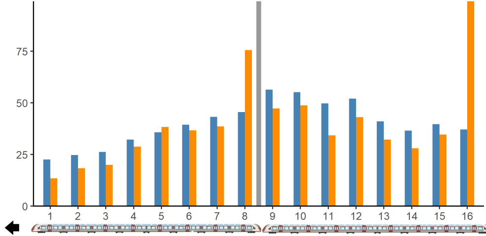
FIGURE 2 – Trajets Paris – banlieue sur la ligne H : diagramme en barres des montées moyennes (en bleu) et des descentes moyennes (en orange) par zones, en nombres de passagers, où les moyennes s’entendent sur l’ensemble des trajets et des gares considérés. La barre grise verticale sépare la rame avant, comportant 8 zones, de la rame arrière, avec elle aussi 8 zones. Les totaux de montées et de descentes moyennes par zones entre les voitures 1 à 8, et 9 à 16, sont égaux : les sommes des hauteurs des barres orange et bleues sont identiques. Dans notre approche, l’estimation des mouvements sera conduite séparément pour chaque rame.
