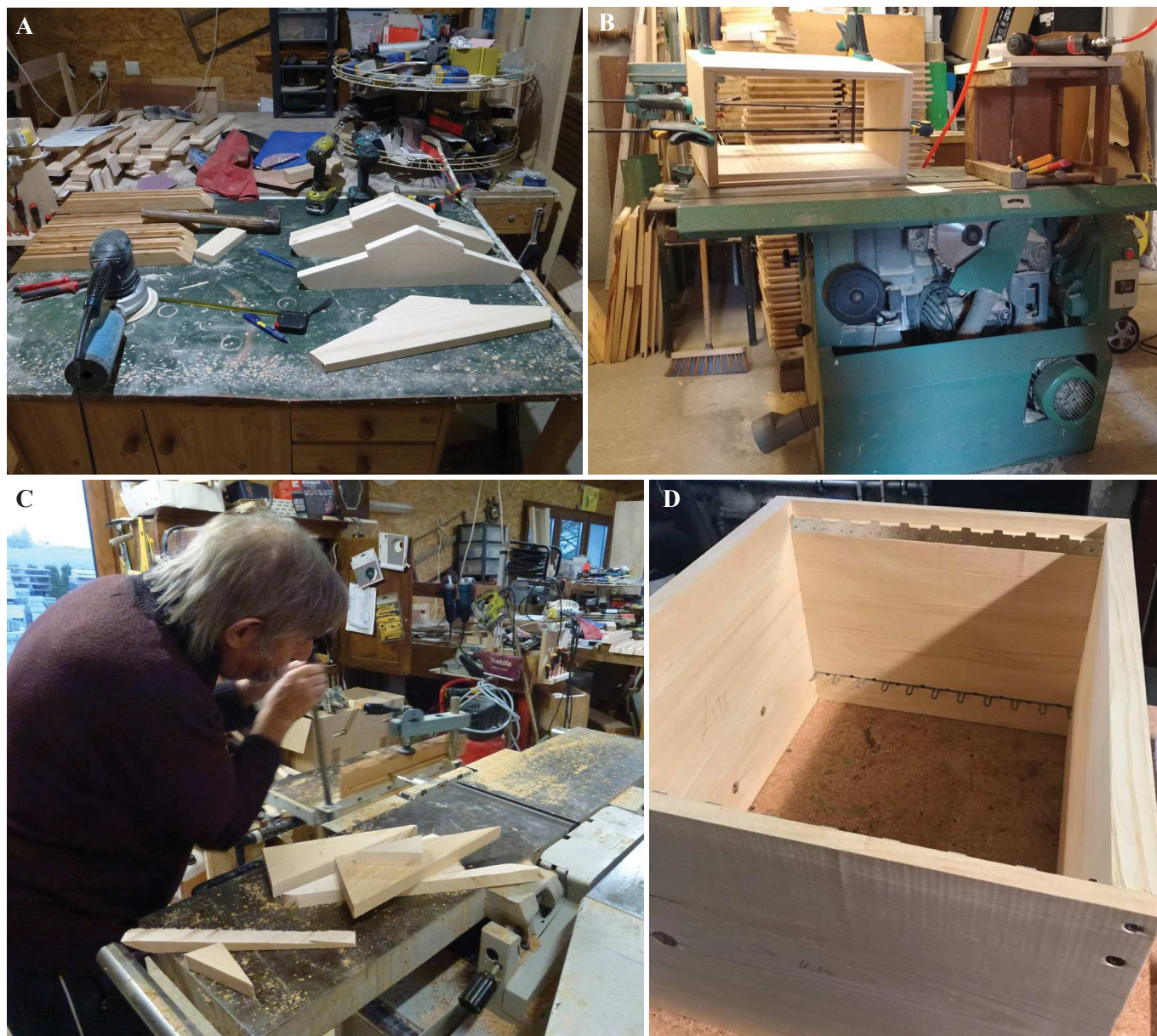
Figure 2. A. Préfabrication des éléments de toits d'une ruche ; B. Montage d'une ruche réalisé au combiné ; C. Passage à la mortaiseuse à mèche pour le rainurage ; D. Exemple de ruche auto-construire. © A. Duplex, D. Humbert.
