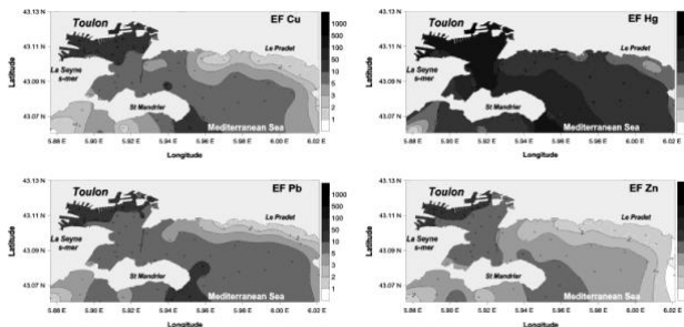
Figure 2 – Distributions spatiales des facteurs d'enrichissement normalisés (Cu, Hg, Pb, Zn) dans la baie de Toulon [6]
