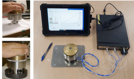
Figure 5: Dispositif portatif d'indentation
