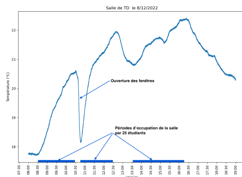
FIGURE 1 – Exemple de relevé de température sur une journée ouverte dans une salle de TD, corrélé à l'occupation.
