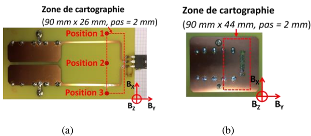
Fig. 6. Prototype de PCB simple face (a) et double face (b)
