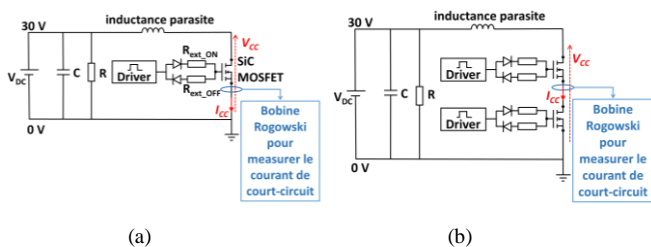
Fig. 7. Schéma électrique du PCB simple face (a) et du PCB double face (b)
