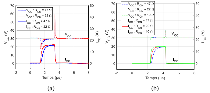
Fig. 8. Formes d'onde de court-circuit testés sur PCB simple face (a) et sur PCB double face (b)
