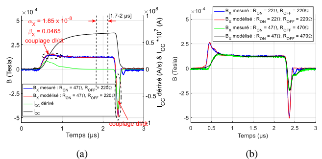
Fig. 9. Réponses impulsionnelles du capteur AMR pour le stress de CC en position 1 sur le PCB simple face à hauteur de 4 mm, avec [R_{ext\_ON}, R_{ext\_OFF}] = [47 \Omega, 220 \Omega] (a), et avec [R_{ext\_ON}, R_{ext\_OFF}] = [22 \Omega, 220 \Omega], [47 \Omega, 470 \Omega] (b).
