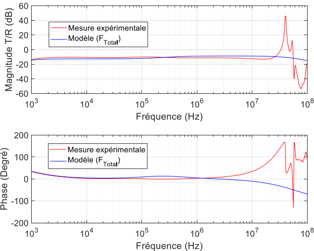
Fig. 15. Comparaison de la fonction de transfert entre la mesure expérimentale et la modélisation du système de capteur à bobine d'induction.
