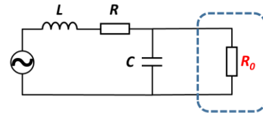
Fig. 3. Circuit équivalent de la bobine d'induction
