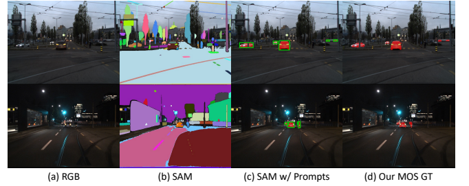
FIGURE 4 : Deux exemples DSEC-MOS [12] : (a) RVB calibrés sur événements; (b) SAM [13] direct; (c) SAM avec des boîtes englobantes de DSEC-MOD; (d) Résultats de segmentation DSEC-MOS, visualisées en rouge sur les images RVB.
