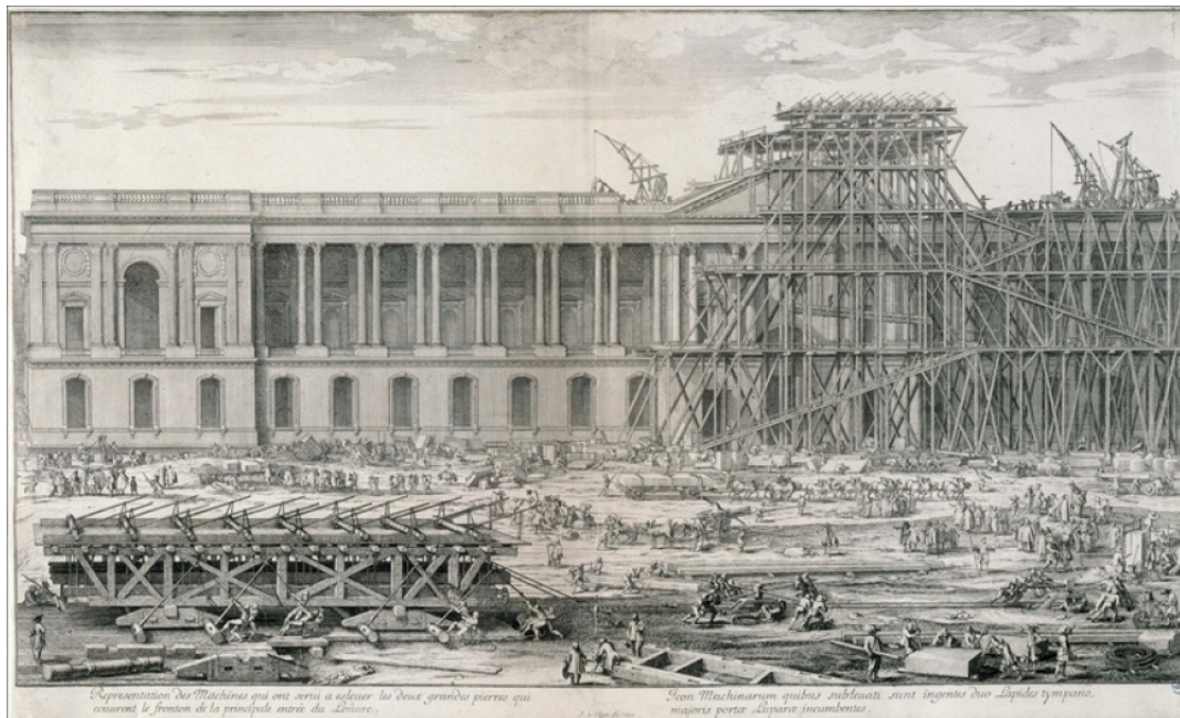
Figure 5 – Sébastien Le Clerc, Représentation des machines qui ont servi à eslever les deux grandes pierres qui couvrent le fronton de la principale entrée du Louvre , 1677, Musée Carnavalet.
