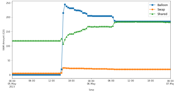
FIGURE 2 – Mémoire balloon et Swap mesurées sur la PM
