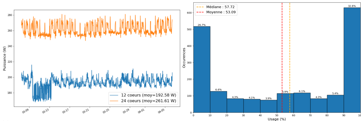
(a) Puissance moyenne sur les serveurs 12 & 24 coeurs de l'infrastructure sur 30 jours
