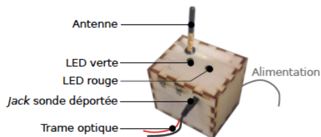
Fig. 8 : Schéma de l'Ensemble de contrôle
