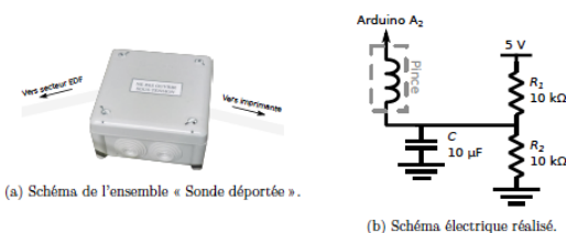
Fig. 7 : Utilisation de la sonde de courant SCT013-005
