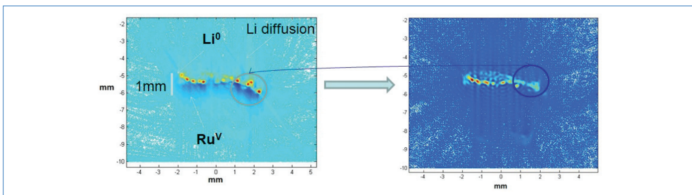
Figure 3 - Les trois méthodes d'Infranalytic peuvent également produire de l'imagerie, notamment dans les cas techniquement complexes des études in situ et in operando . La RPE permet ici de localiser les ions RuV en charge sur une électrode de 1 mm, dans une batterie lithium-ion en fonctionnement, de constater leur transformation et de mesurer la formation d'agrégats de lithium diffusant au cours des cycles de charge, induisant une diminution des performances des batteries. (Photo M. Sathiya., J.-B. Leriche, E. Salager, D. Gourier, J.-M. Tarascon, H. Vezin).
