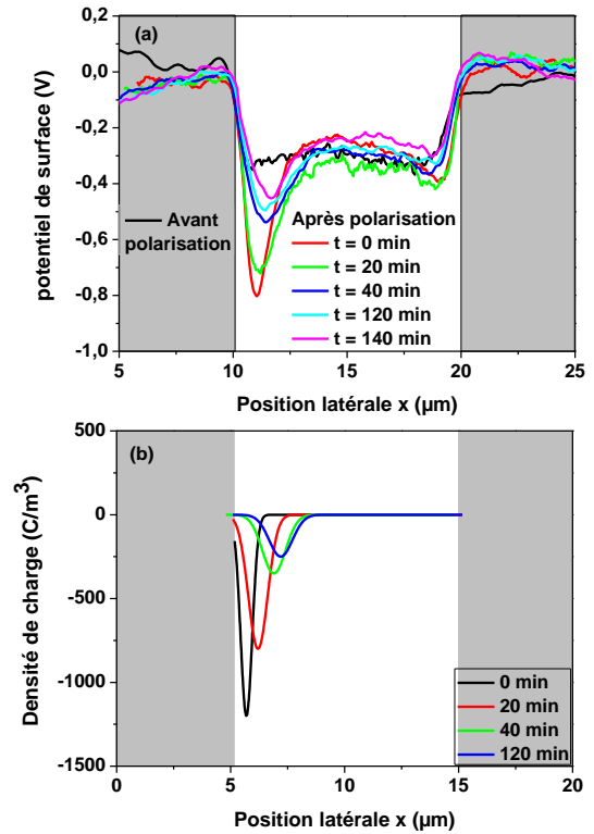
Fig. 4. Evolution au cours du temps, après polarisation pendant 1 h sous 20 V (a) du profil de potentiel de surface mesuré par FM-KPFM et (b) de la densité de charge d'espace.
