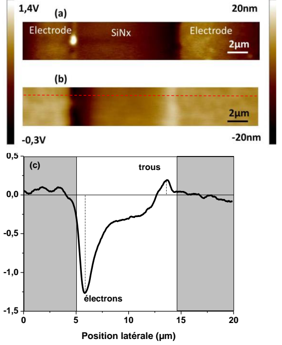
Fig. 2. Cartographies de (a) topographie et (b) de potentiel de surface mesurées par FM-KPFM après une polarisation de 1 h sous 40 V. (c) Profil de potentiel pris au niveau de la ligne en pointillés rouge.
