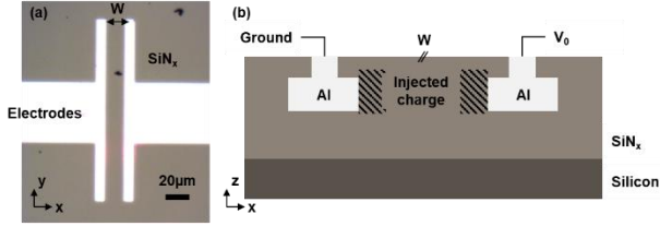
Fig. 1. (a) Vue de dessus, au microscope optique, de la structure MIM. (b) Schéma vu en coupe de la structure MIM.
