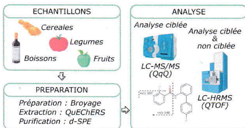
Figure 3. Schéma de la méthodologie analytique envisagée dans le projet de recherche.
