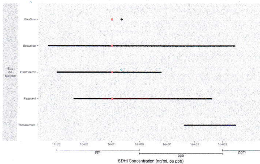
Figure 2. Gamme de concentration en SDHI mesurée dans des eaux de surface et limites de qualité française des eaux de consommation humaine (point rouge). Echelle logarithmique des concentrations.
