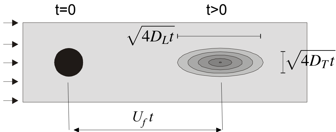
Figure 6. Illustration de la dispersion d'un panache de polluant
