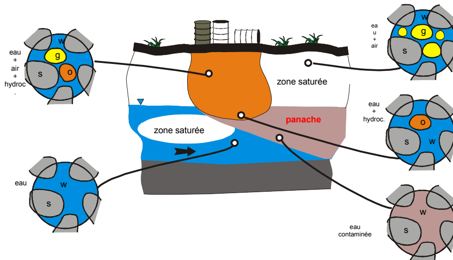
Figure 3. Schéma d'une nappe aquifère polluée
