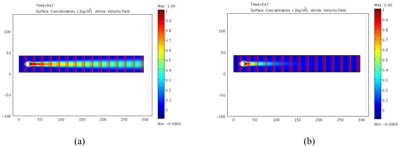
Figure 10. Panache de polluant développé derrière une zone source (cercle blanc sur la figure) : (a) transport, dilution et dispersion, (b) mêmes mécanismes avec en outre de la biodégradation
