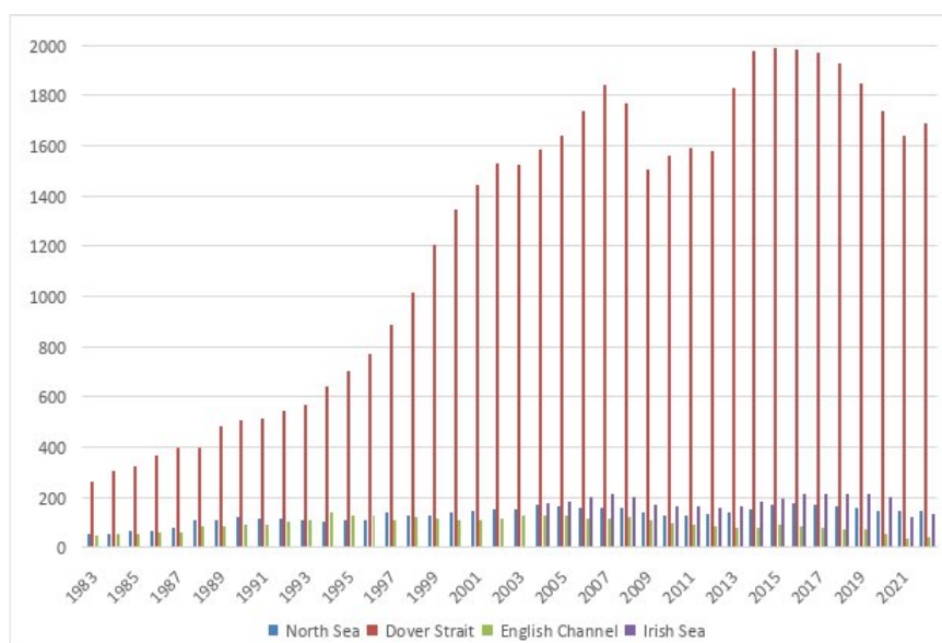
Graphique 2. Trafic de fret entre le Royaume-Uni et le continent (y compris tunnel sous la Manche) par zones maritimes de 1983 à 2022, en milliers de remorques accompagnées.
