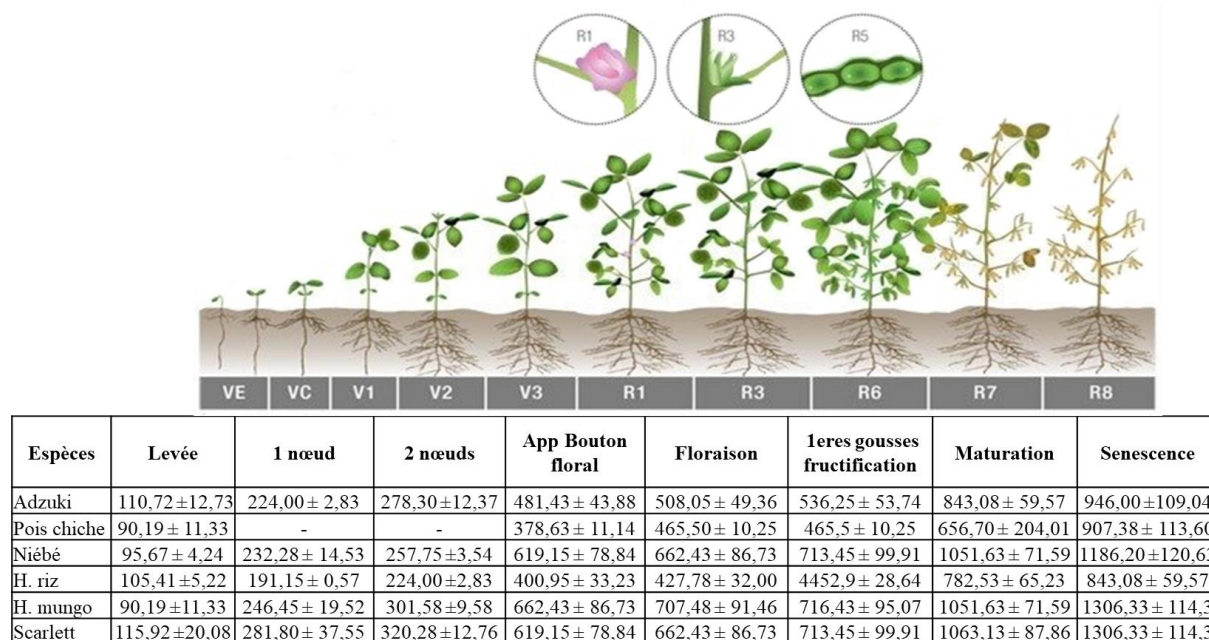
Figure 1 : Moyenne de la somme de températures (°CJ 1 ) nécessaire pour atteindre les différents stades de développement de chaque espèce. Calculés sur des plantes cultivées sous différentes conditions thermiques. Avec une température de base de 10°C (photo : http://blog.agriconomie.com/le-pois-et-le-soja/2014 ).
