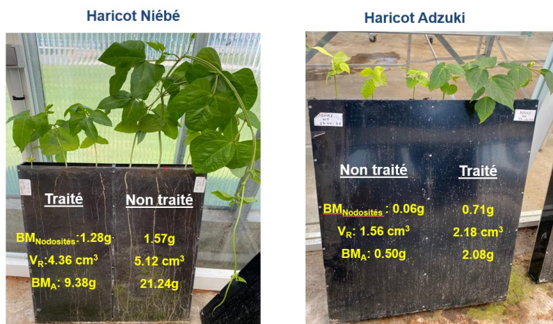
Figure 4 : Impact de l'inoculation avec Bradyrhizobium japonicum G49 sur la croissance aérienne ( BM_A ), sur le volume racinaire ( V_R ) et sur la biomasse de nodules produits ( BM_{\text{Nod}} )
