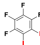
1,2TFIB
