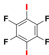
1,4TFIB
