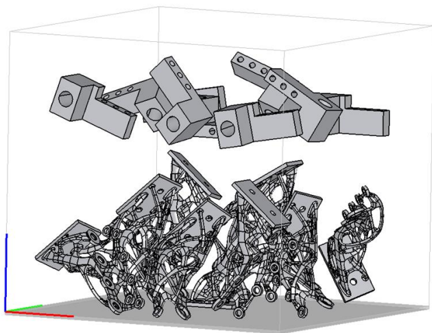
Figure 6 – Positionnement des pièces dans la machine EBM
