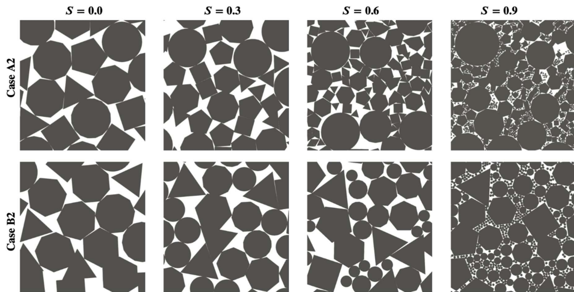
Figure 5. Échantillons pour le cas A2 (en haut) et le cas B2 (en bas) pour les plages de taille de particule S=0,0 , S=0,3 , S=0,6 et S=0,9 .
