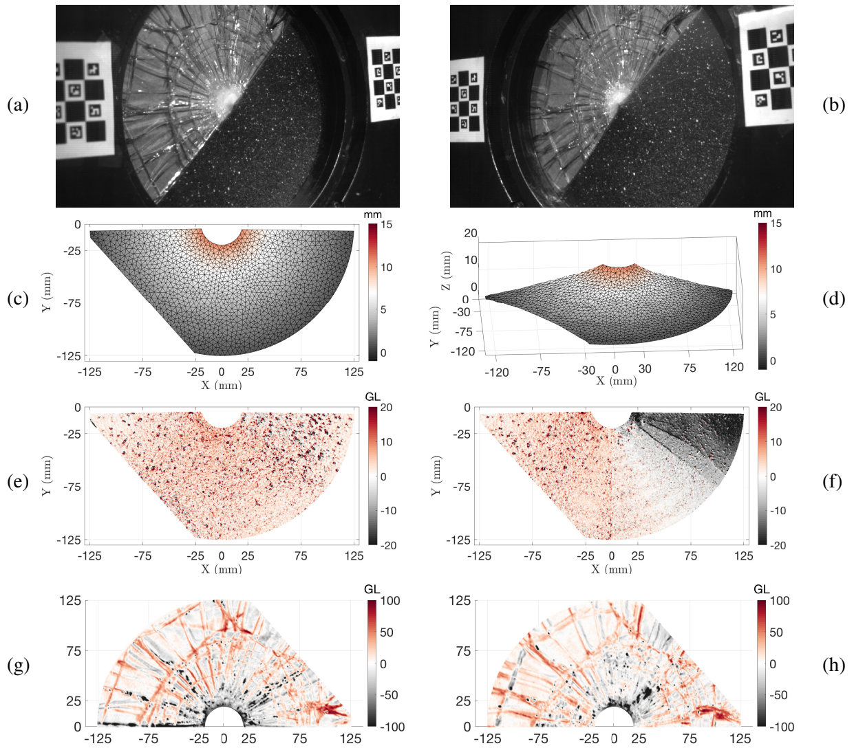
FIGURE 5 – Mesures par S-CIN axisymétrique à t=1.63 ms ( i.e. image 50) : (a)-(b) Images stéréo. Déplacement hors-plan sur la surface de référence (c) et déformée (d). Les résidus de corrélation d'images (e)-(f). Les résidus de la zone non-mouchetée pour la lecture de la fissuration (g)-(h).
