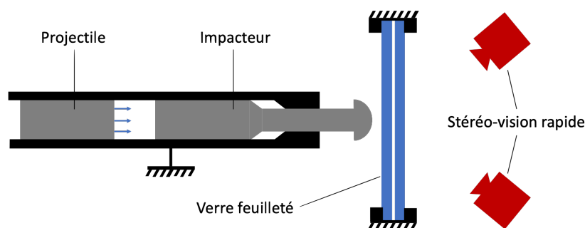
FIGURE 1 – Schéma du système "canon".
