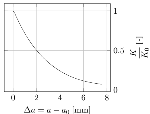
FIGURE 4 – Perte de raideur en fonction de l'incrément de longueur de fissure, simulée par éléments finis via l'ouverture des noeuds sur le chemin de fissure.
