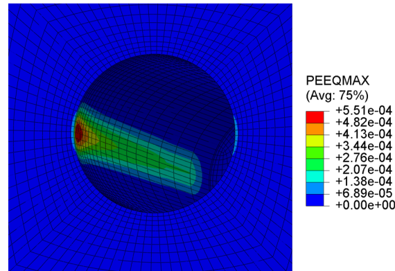
FIGURE 2 – : Déformation plastique équivalente, suite à une précharge de 6000 N et un déplacement de 50 \mu\text{m}
