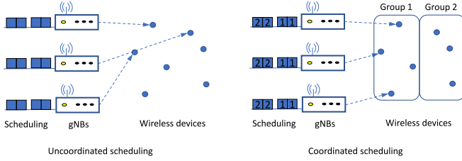
Fig. 4: Scheduling scenarios.
