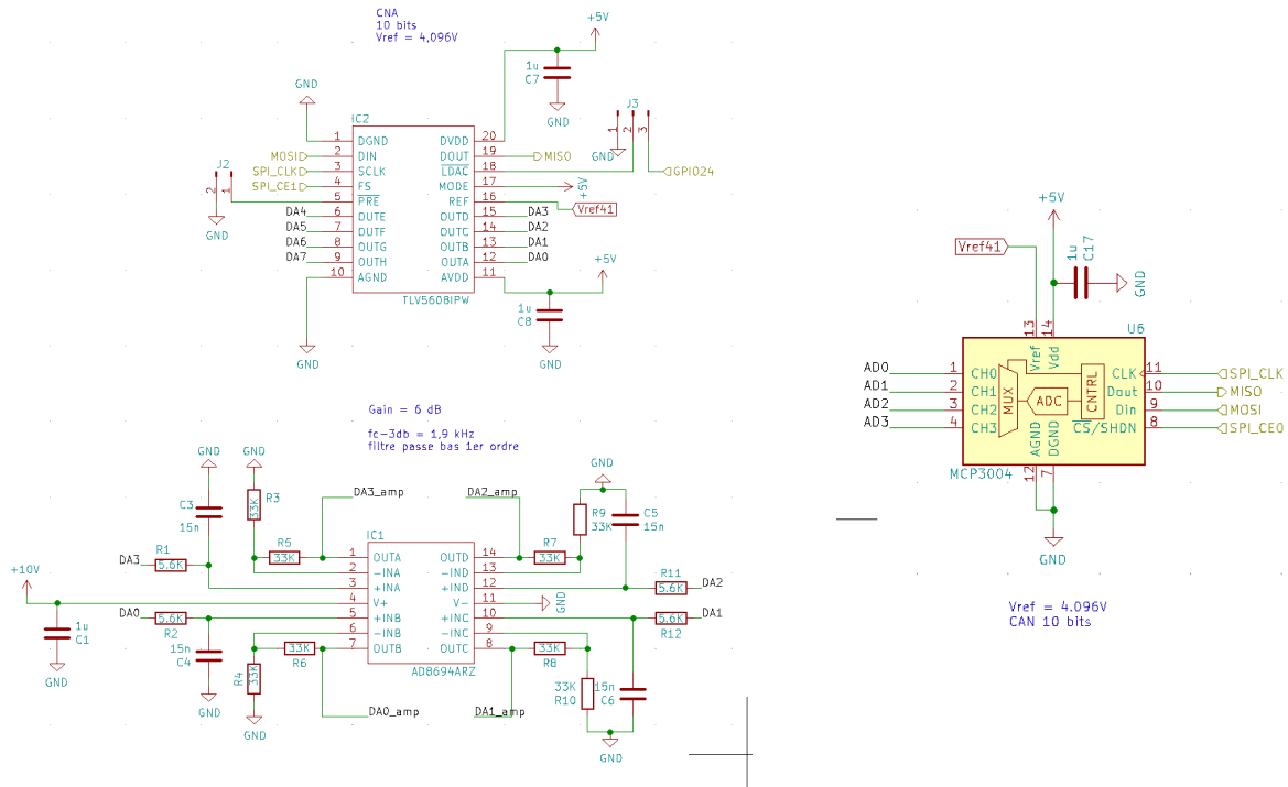
Fig 16 : Extrait du schéma de la carte d'interface
