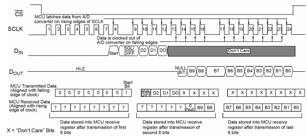
Fig 14 : Trame SPI lecture données
