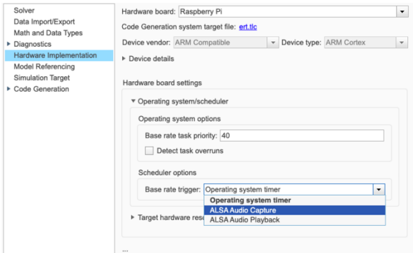
Fig 22 : Paramètres de l'OS/Scheduler
