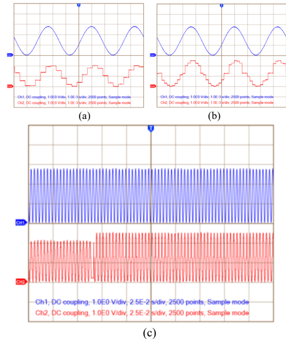
Fig 21 : Oscillogramme pour différentes périodes d'échantillonnage
