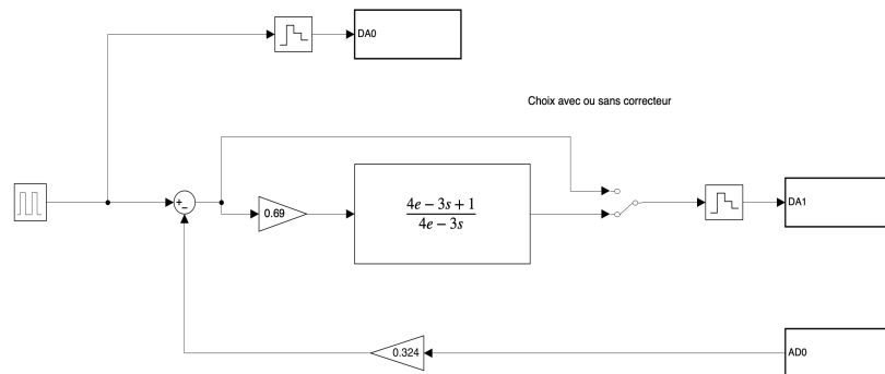
Fig 17 : Régulateur PI pour l'alimentation à découpage
