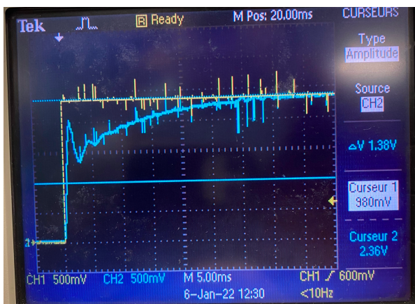
Fig 19 : Réponse du système en BF avec correcteur PI
