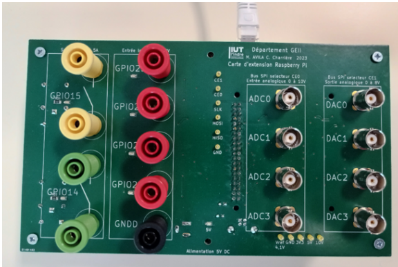
Fig 15 : PCB de la carte d'interface
