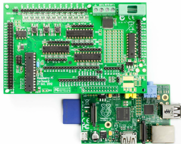
Fig 10 : Vue de la carte Gertboard
