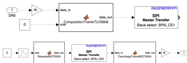
Fig 12 : Bloc de gestion des entrées et sorties analogiques
