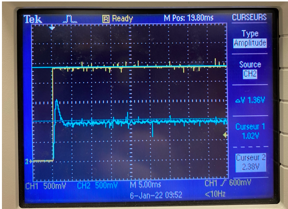
Fig 18 : Réponse du système en BF sans correcteur
