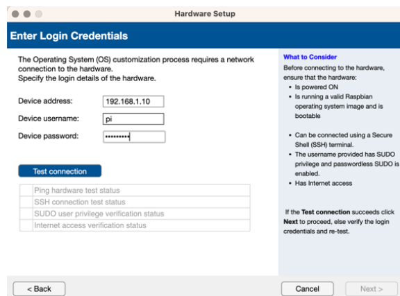
Fig 5 : Personnalisation d'un OS existant
