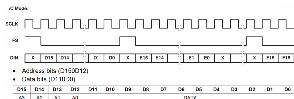
Fig 13 : Trame SPI à envoyer
