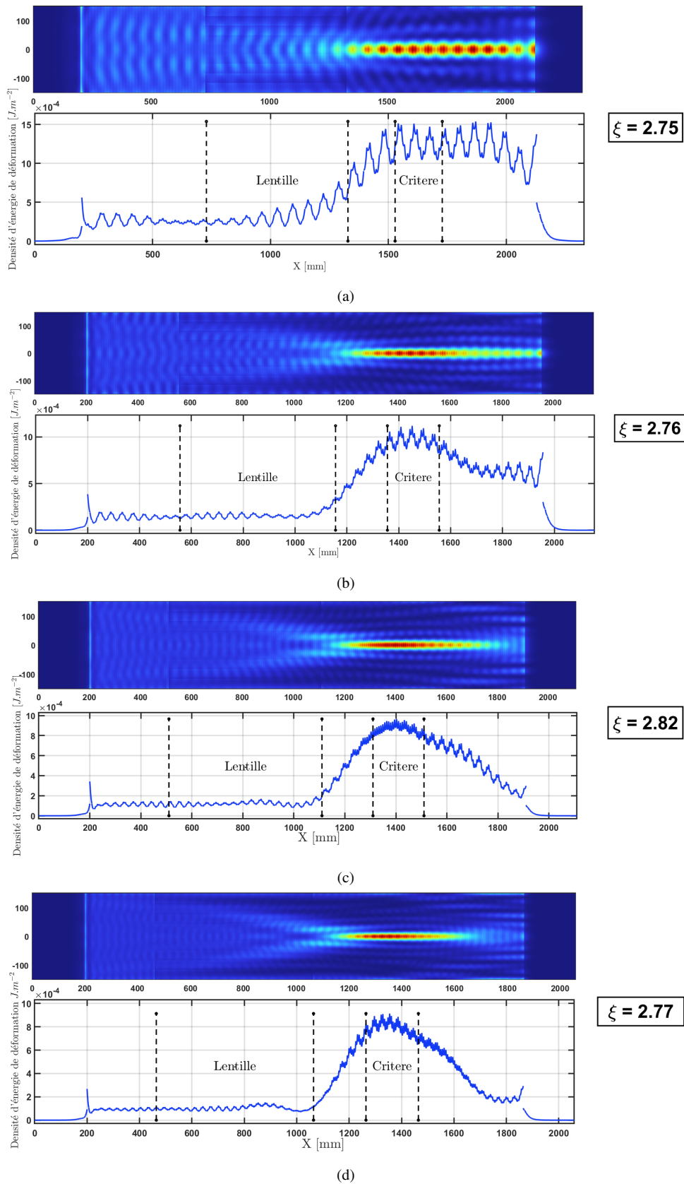
FIG. 9. – Répartition de l'énergie de déformation suivant le plan (\vec{x}, \vec{y}) de la plaque, densité d'énergie de déformation suivant l'axe de symétrie (central) de la structure lentille et valeur du critère de performance \xi pour la configuration décrite par (Tab. 1) pour les fréquences suivantes : (a) f = 2000 Hz, (b) f = 4400 Hz, (c) f = 5800 Hz et (d) f = 8000 Hz
