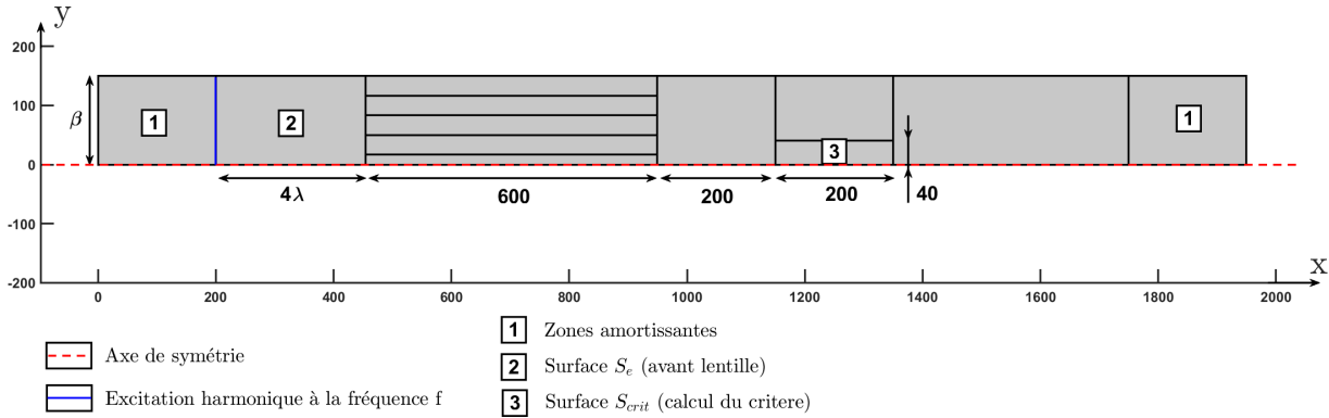
FIG. 8. – Géométrie du modèle numérique de la structure lentille correspondant aux paramètres définis dans la partie 4.1 pour f = 8000\text{Hz} , (dimensions en mm)
