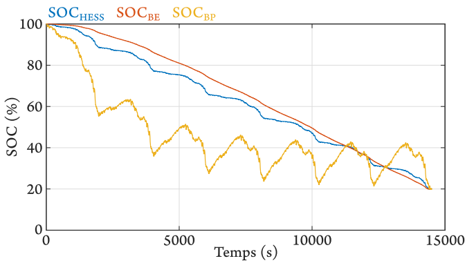
Fig. 8. Évolution des SOC du couple Panasonic – A123.
