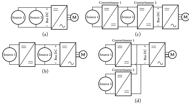
Fig. 1. Architectures classiques de couplage : (a) Connexion directe, (b) Architecture cascade à 1 convertisseur DC-DC, (c) Architecture cascade à 2 convertisseurs DC-DC, (d) Architecture parallèle, (adaptée de [6]).
