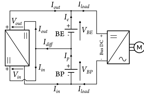
Fig. 3. Architecture série.
