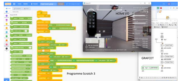
fig 7 : La commande du garage en Scratch 3
