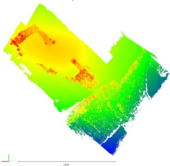
Fig. 9 - ANR Monumen – mission des 15-17/03/2021 – Marcoux – Tous les points lidar
