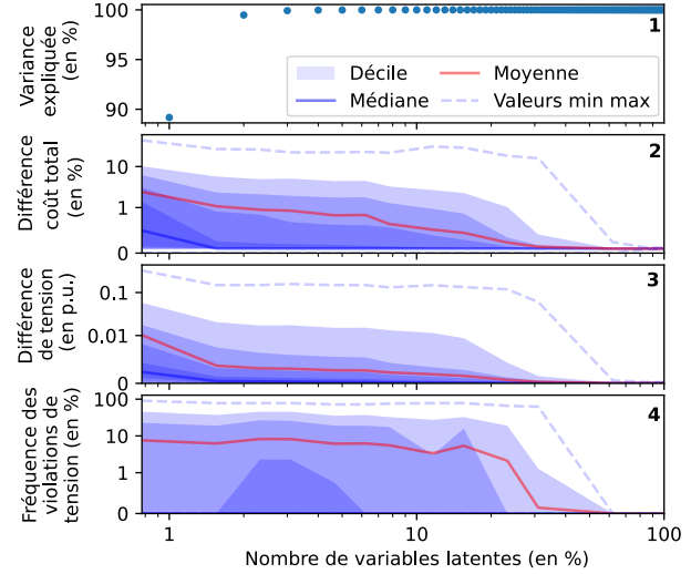
FIG. 3. Effet de la réduction de dimension sur la sous-optimalité du contrôle. Le panneau 1 représente l'information contenue dans chaque composante de la représentation latente. Les panneaux suivants représentent différents écarts |E - \tilde{E}| entre la stratégie OPF et la stratégie proposée en fonction du nombre de composantes conservées dans l'espace latent (étape 5). Les panneaux 2 et 3 représentent respectivement les écarts de coûts et du plan de tension. Le panneau 5 décrit la fréquence des violations de tension.
