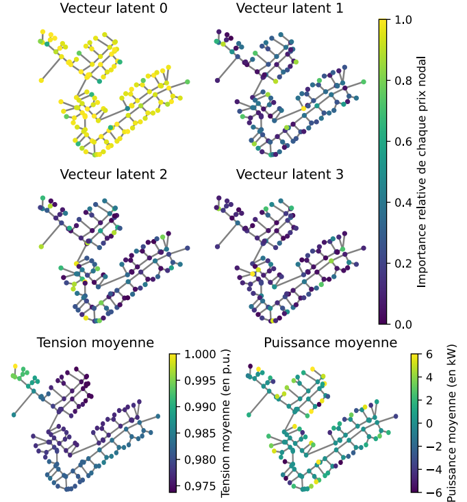
FIG. 5. Analyse des vecteurs propres de la matrice ACP via l'emplacement de chaque prix nodal sur le réseau. Les quatre premiers vecteurs latents sont représentés. Les contributions de chaque prix nodal sont normées de sorte que l'importance maximale pour chaque vecteur soit égale à 1. La figure représente également la tension moyenne et la puissance moyenne observée sur chaque bus lors de la simulation.
