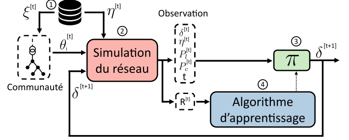
FIG. 3. Apprentissage par renforcement du coût d'utilisation de la ligne. ① Les variables exogènes à l'instant t – noté \xi^{[t]} – issues d'une base de données sont transmises à la communauté énergétique qui donne en retour les prix \theta_i^{[t]} de chaque acteur. ② Ces prix \theta_i^{[t]} , accompagnés du prix du réseau \eta^{[t]} et du coût d'utilisation de la ligne \delta^{[t]} permettent de calculer l'ordre de mérite et d'en déduire le vecteur d'observation O^{[t]} . ③ L'observation est transmise au GR pour qu'il déduise le prochain prix \delta^{[t+1]} . ④ En parallèle, un algorithme d'apprentissage améliore les performances du contrôleur grâce à un signal de récompense pénalisant les violations des contraintes.
