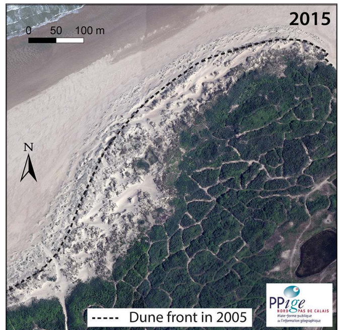
Fig. 8 – Photographies aériennes montrant la progression vers la mer du champ de dunes embryonnaires de 2005 à 2015.
