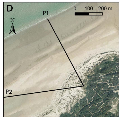
Fig. 9 – Profils topographiques DGPS de la plage et des dunes côtières à l'est de Calais.
