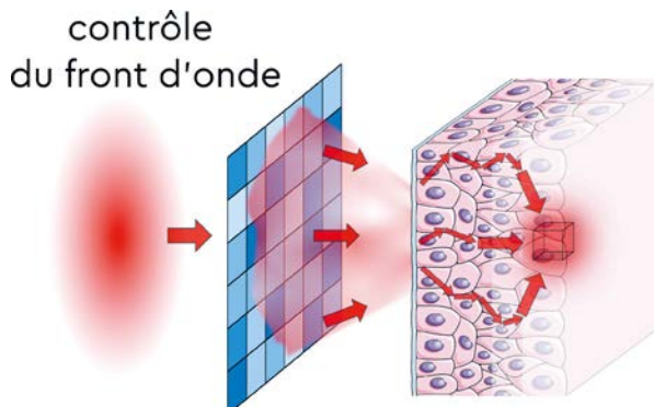
Figure 3 : Concept de la focalisation en profondeur. Il est nécessaire d'avoir une «étoile-guide» non-invasive pour pouvoir guider la lumière en profondeur. De multiples méthodes (utilisant l'acoustique ou la fluorescence) ont été proposées.
