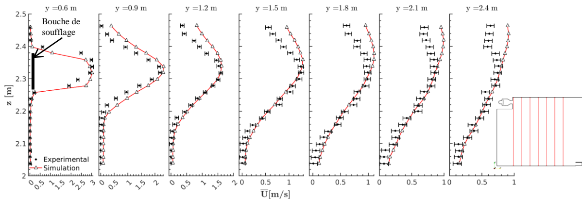
Figure 4 : Profils de vitesse moyenne dans le plan median
