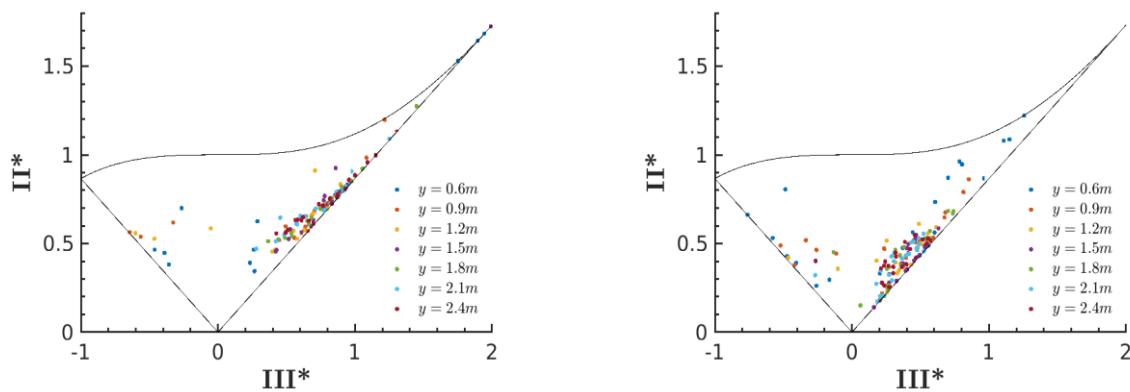
Figure 7 : Triangles de Lumley, expérimental (à gauche) et simulé (à droite)
