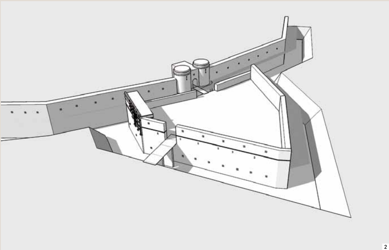
1 - Visualisation en 3D du boulevard de Louis XI © David Leclercq (AUAP) 2 - Visualisation en 3D du boulevard de François 1 er © David Leclercq (AUAP)
