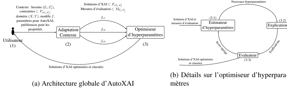
FIG. 1 – Architecture d'AutoXAI.
