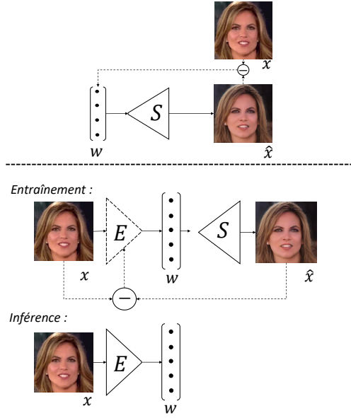
FIGURE 1 : Les deux méthodes principales de l'inversion de StyleGAN, les flèches en pointillés désignent respectivement le procédé d'optimisation et l'apprentissage de l'encodeur. Le réseau de synthèse de StyleGAN est représenté par le bloc S . En haut, la méthode par optimisation fournit un code w optimisé en minimisant une différence dans l'espace image jusqu'à obtention d'un résultat satisfaisant. En bas, un réseau encodeur E est entraîné à fournir directement à partir de l'image un code qui permet de reconstruire l'image. Le processus d'inférence est représenté simplement en dessous.
