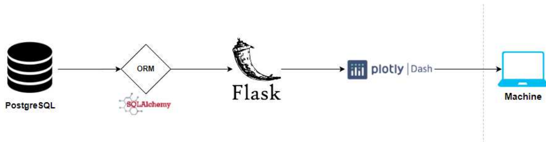
Figure 4:1 Architecture du système côté API
